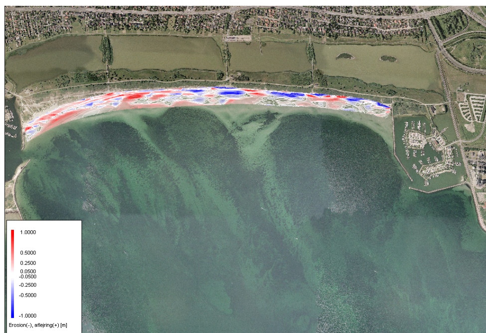
Figur 9.0 Erosion og aflejring fra 2002 til 2007
